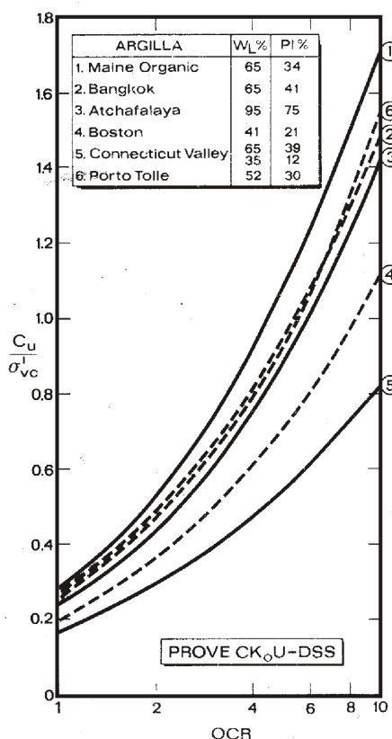
Fig. 7.3 – Variazione della C_u (coesione non drenata) con OCR (grado di sovraconsolidazione) per terreni coesivi (LADD & EDGERS, 1972).
