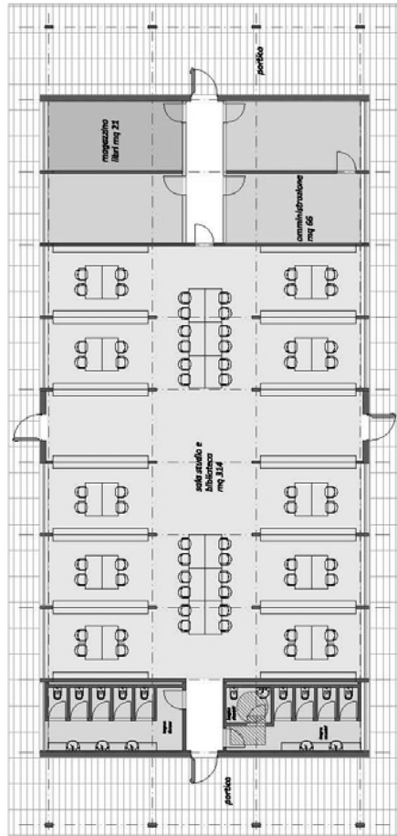
BIBLIOTECA E AREE STUDIO piano terra
