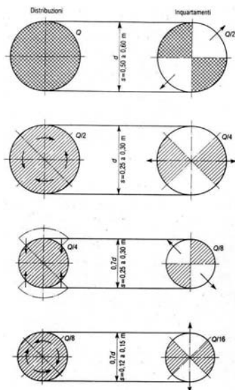
Figura 1 – schema di riduzione per quartatura
